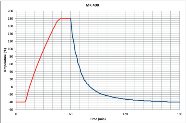
Aufheizkurve / Abkühlkurven
