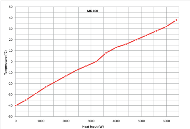
Wärmekompensationsdiagramm
