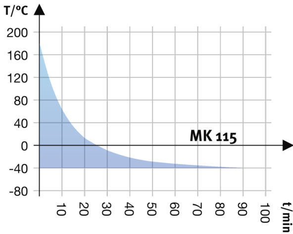
Abkühlkurve
